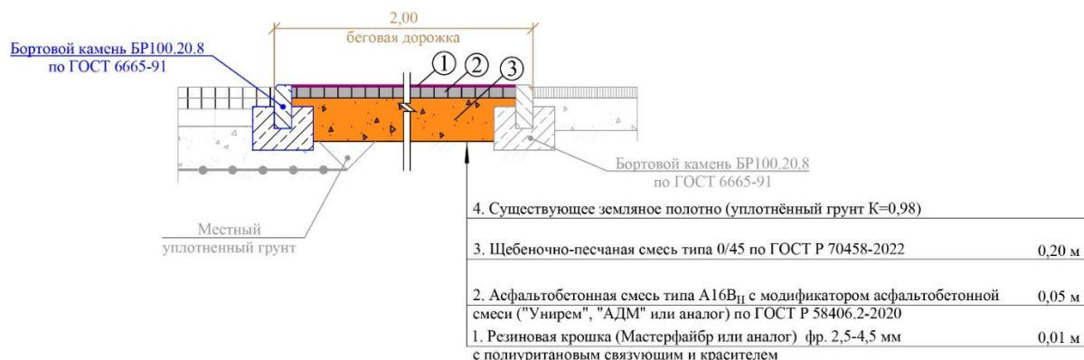
Рис. 28. Конструкция дорожной одежды. Тип 2 (укладывается на беговой дорожке)
