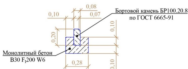
Рис. 29. Конструкция дорожной одежды. Тип 2 (укладывается на беговой дорожке)
