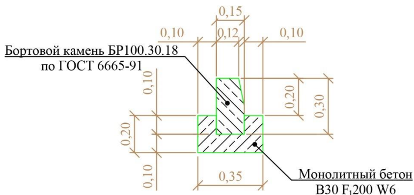
Рис.26 Конструкция дорожной одежды. Тип 1 (укладывается по территории и вокруг стадиона)
