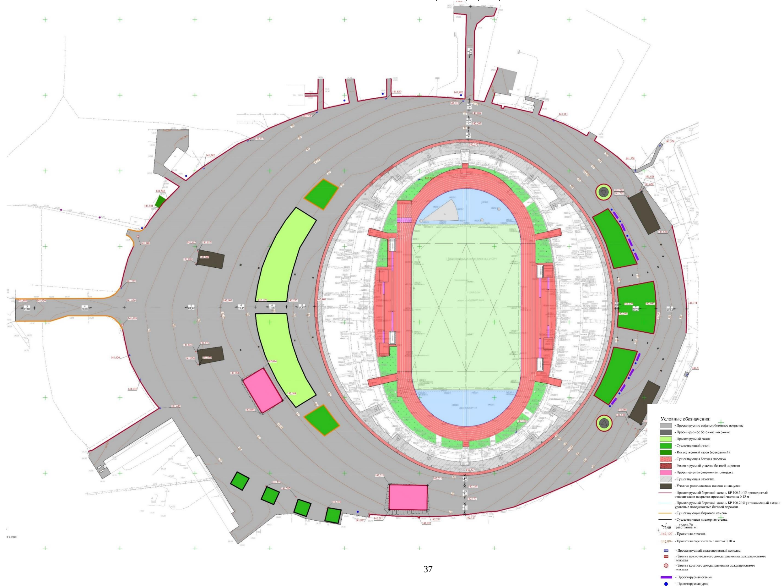
Рис.24. Схема организации рельефа
