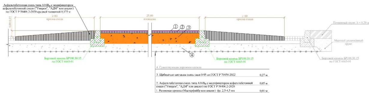
Рис.30. Конструкция дорожной одежды. Тип 3 (укладывается на спортивной площадке)
