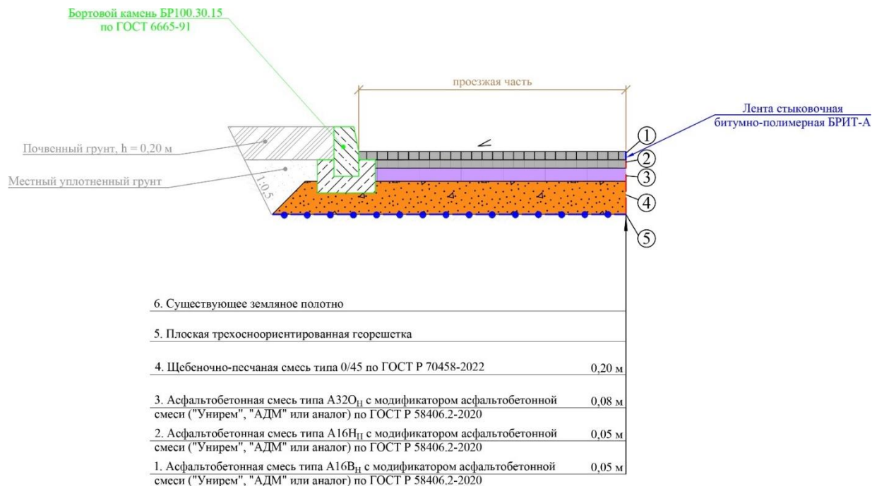
Рис.25 Конструкция дорожной одежды. Тип 1 (укладывается по территории и вокруг стадиона)
